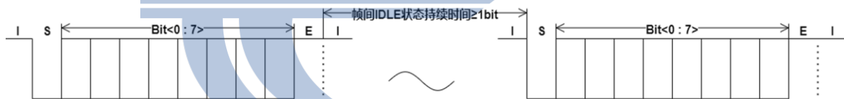
图9 数据帧间时序要求
