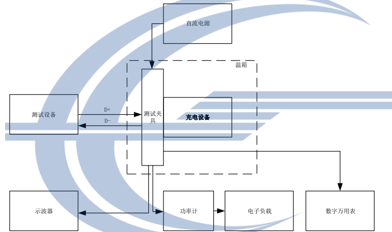
图2 充电设备测试推荐组网图
