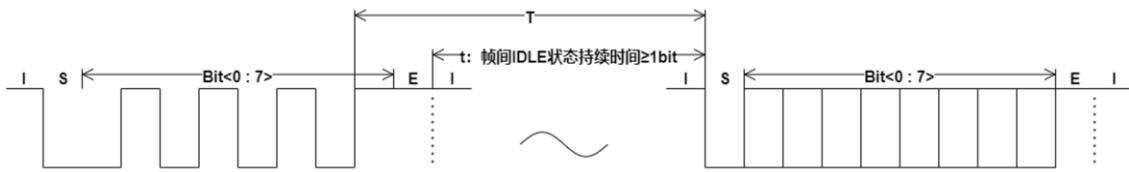
图8 数据帧间高电平持续时间 T 和 idle 状态持续时间 t
